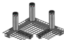
Esempio di posa angolare (angolo 90°)
